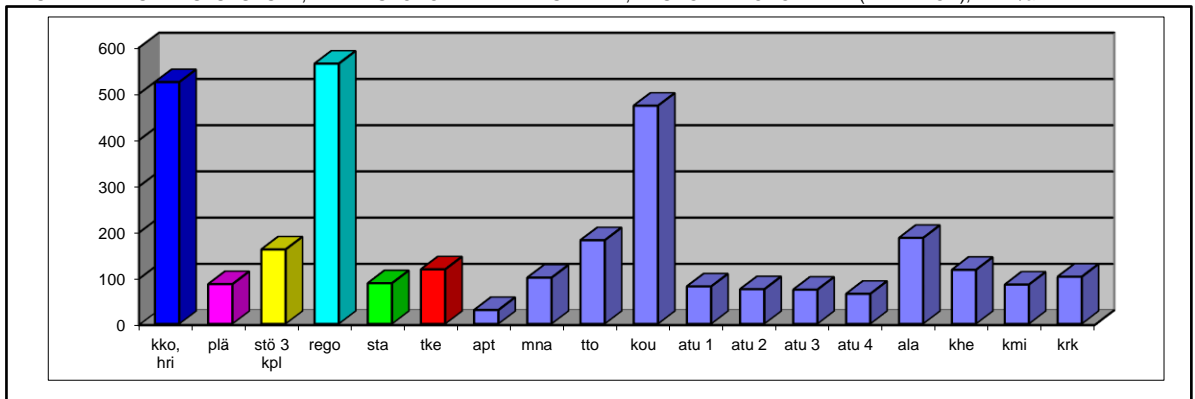
KAAVIO 2.1 LASKENNALLISET KULUTUKSET, KIINTEISTÖKOHTAINEN LASKENTA, KAUKOLÄMPÖKOHTEET (NYKY POK), MWh/a
