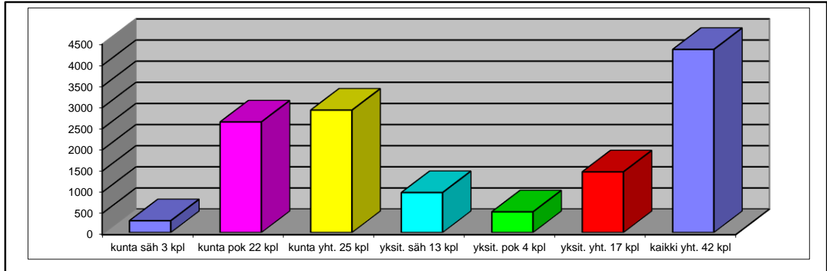
KAAVIO 1.1 LASKENNALLISET KULUTUKSET, MASSALASKENTA, MWh/a
